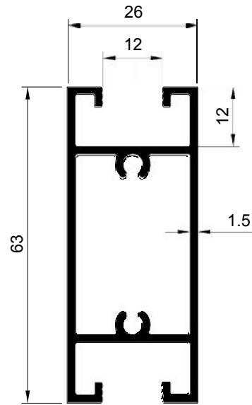
SECTION NO. - 80S-2801 EST. WEIGHT - 0.908 KG./M.
