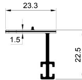
SECTION NO. - 80SFL-1001 EST. WEIGHT - 0.224 KG./M.
