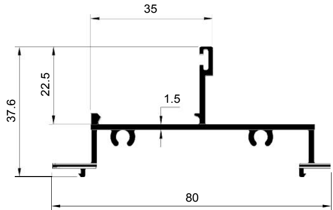
SECTION NO. - 80SFL-1004 EST. WEIGHT - 0.660 KG./M.
