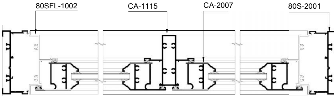
SECTION :- E - E
