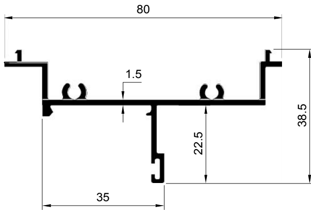
SECTION NO. - 80SFL-1002 EST. WEIGHT - 0.655 KG./M.
