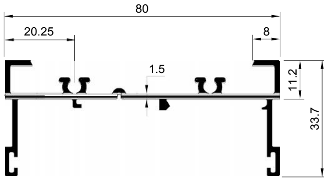
SECTION NO. - 80S-2001 EST. WEIGHT - 0.821 KG./M.
