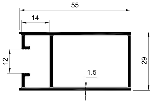
SECTION NO. - 80S-2701 EST. WEIGHT - 0.723 KG./M.
