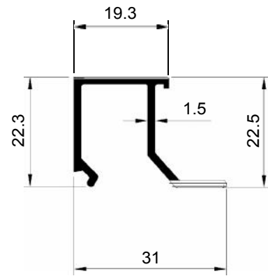
SECTION NO. - GL-110 EST. WEIGHT - 0.305 KG./M.
