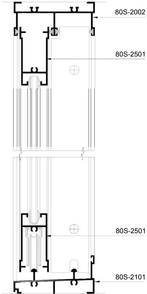
SECTION:- A-A
