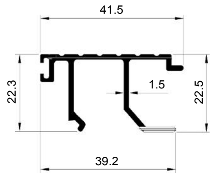
SECTION NO. - GL-111 EST. WEIGHT - 0.435 KG./M.
