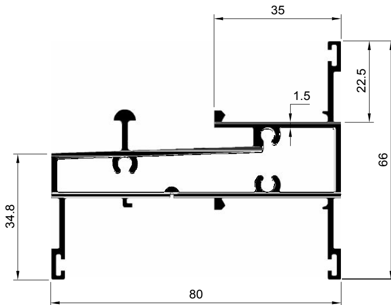
SECTION NO. - 80S-2302 EST. WEIGHT - 1.423 KG./M.
