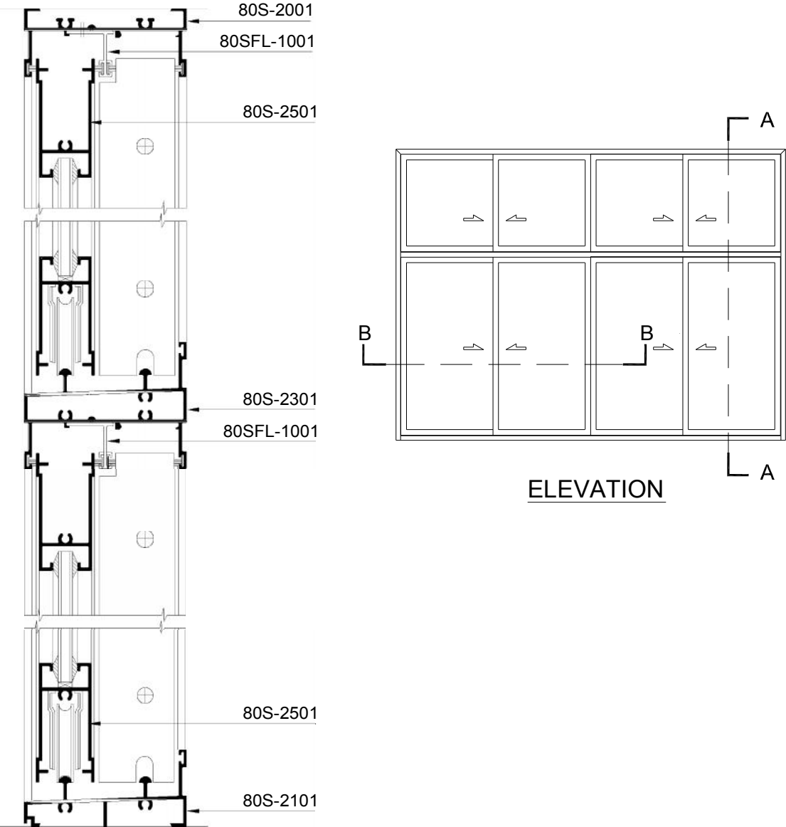
SECTION:- A-A
