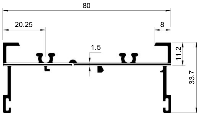
SECTION NO. - 80S-2001 EST. WEIGHT - 0.821 KG./M.
