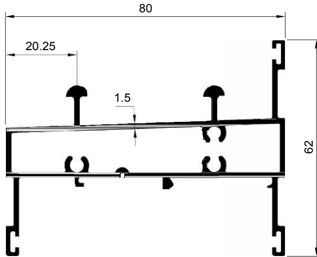
SECTION NO. - 80S-2301 EST. WEIGHT - 1.390 KG./M.
