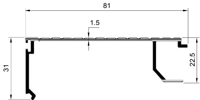
SECTION NO. - GL-112 EST. WEIGHT - 0.588 KG./M.
