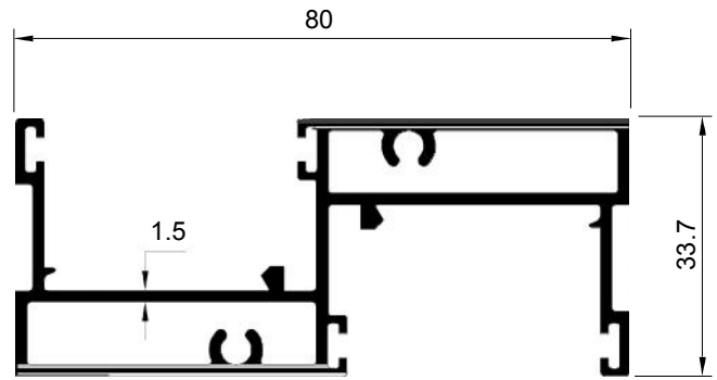
SECTION NO. - 80S-2201 EST. WEIGHT - 1.237 KG./M.
