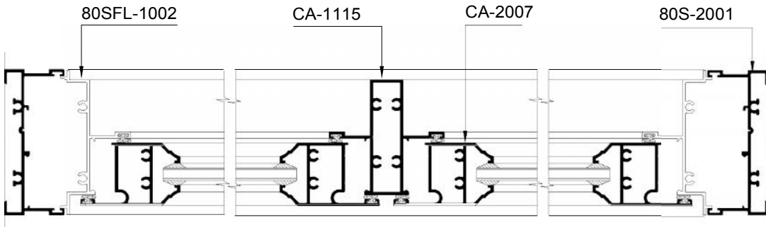
SECTION :- E - E
