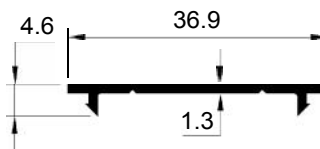
SECTION NO. - HDR-104 EST. WEIGHT - 0.148 KG./M.
