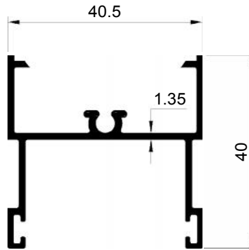
SECTION NO. - SS-2001 EST. WEIGHT - 0.544 KG./M.
