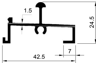
SECTION NO. - SS-2101 EST. WEIGHT - 0.427 KG./M.
