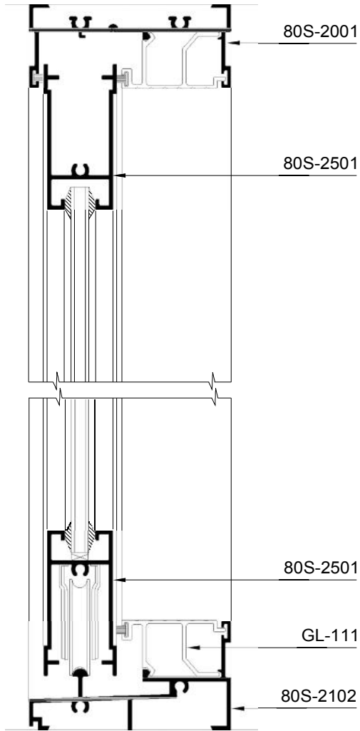
SECTION:- A-A
